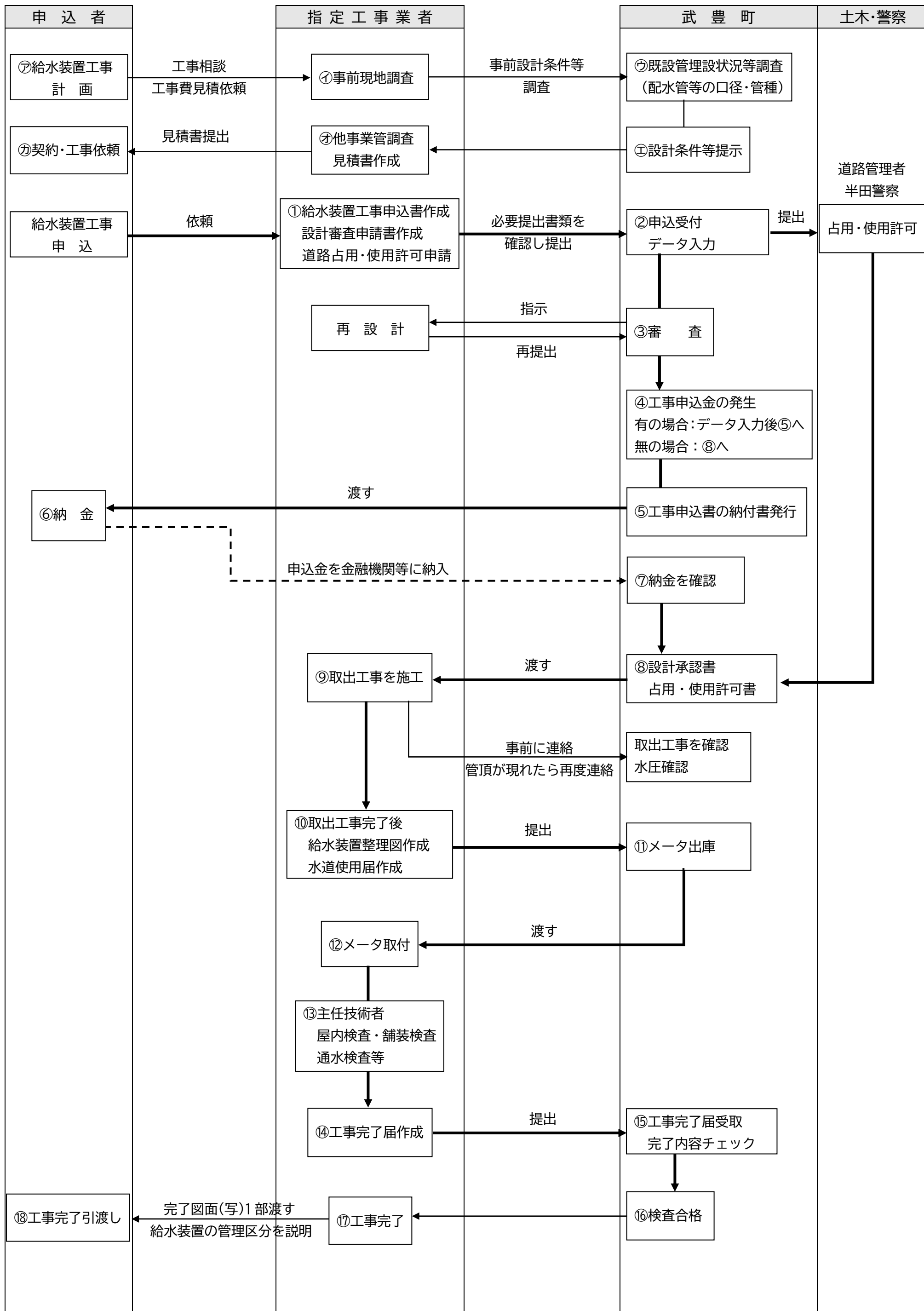
給水装置工事フローチャート（標準）
